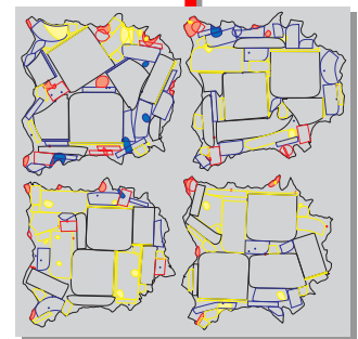
multineest
